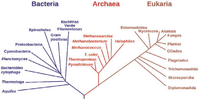
Figura 6.6. Árvore filogenética da biodiversidade terrestre, mostrando os três grandes reinos ( Bacteria , Archaea e Eukarya ), todos ligados a uma raiz comum (Pace, 1997) (Creative Commons)
