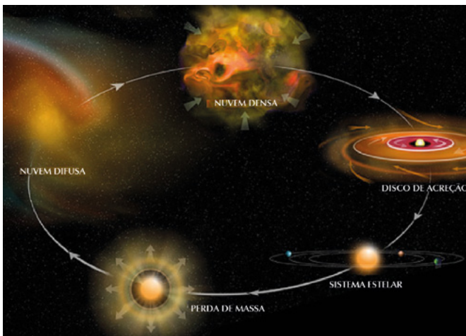
Figura 4.2. As fases do processo de formação planetária. Fonte: Adaptado de Harvard Smithsonian Center for Astrophysics (CfA)
