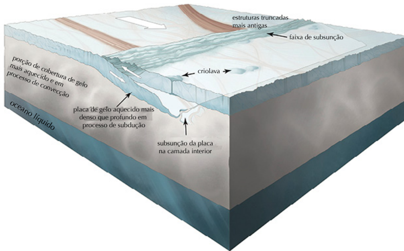
Figura 12.8. Representação do processo de subducção entre placas tectônicas em Europa. Fonte: Nasa/Noah Kroese, I.NK
