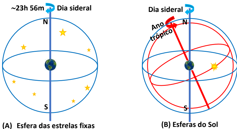
Figura 16. Modelo de Eudoxo
