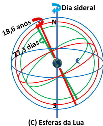
(C) Esferas da Lua
